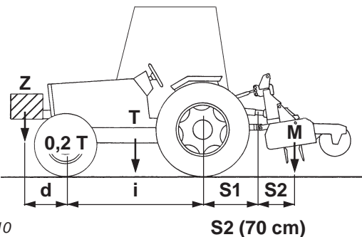
Macchina in manovra nel campo Machine manoeuvring in the field Maschine im Manöver auf dem Feld Machine en manœuvre sur champ Máquina en maniobra en el campo
