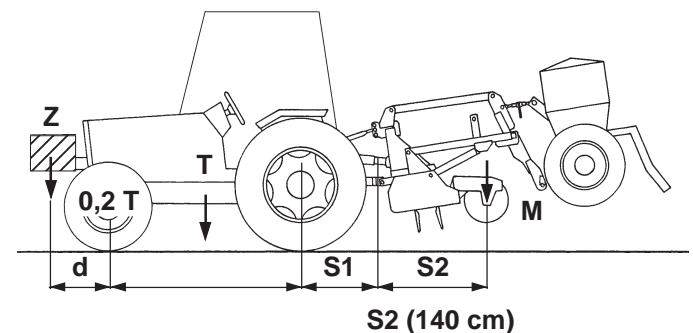
Macchina con attacco e seminatrice a sbalzo in manovra nel campo Machine with hitch and overhanging seed drill manoeuvring in the field Maschine mit Kupplung und überstehender Drillmaschine im Manöver auf dem Feld Machine avec attelage et semoir déporté en manœuvre sur champ Máquina con enganche y sembradora saliente en maniobra en el campo
