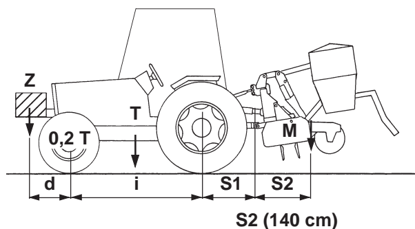
Macchina con seminatrice in manovra nel campo Machine with seed drill manoeuvring in the field Maschine mit Drillmaschine im Manöver auf dem Feld Machine avec semoir en manœuvre sur champ Máquina con sembradora en maniobra en el campo
